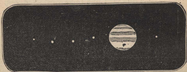
Júpiter con sus satélites.
